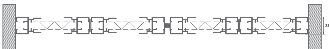
SEZIONE ORIZZONTALE 4 ANTE
