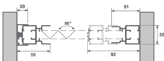
SEZIONE ORIZZONTALE 2 ANTE
