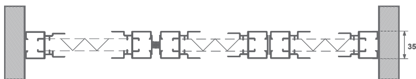
SEZIONE ORIZZONTALE 3 ANTE
