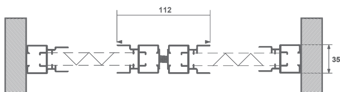
SEZIONE ORIZZONTALE 1 ANTA
